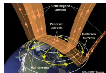
図3 地球極域の沿磁力線電流
