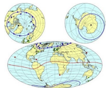
図2 地上の磁場観測網
