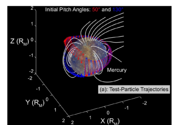
図4 荷電粒子の軌道
