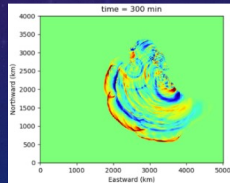
津波伝播
